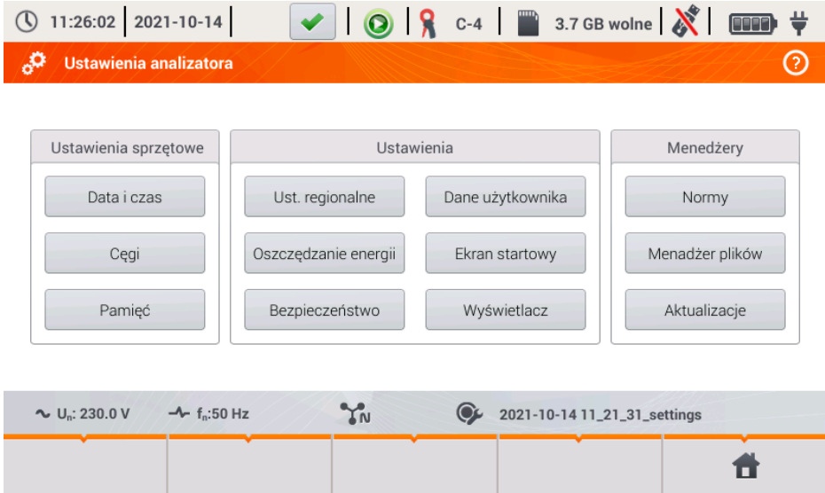
Rys. 15. Ustawienia analizatora.
